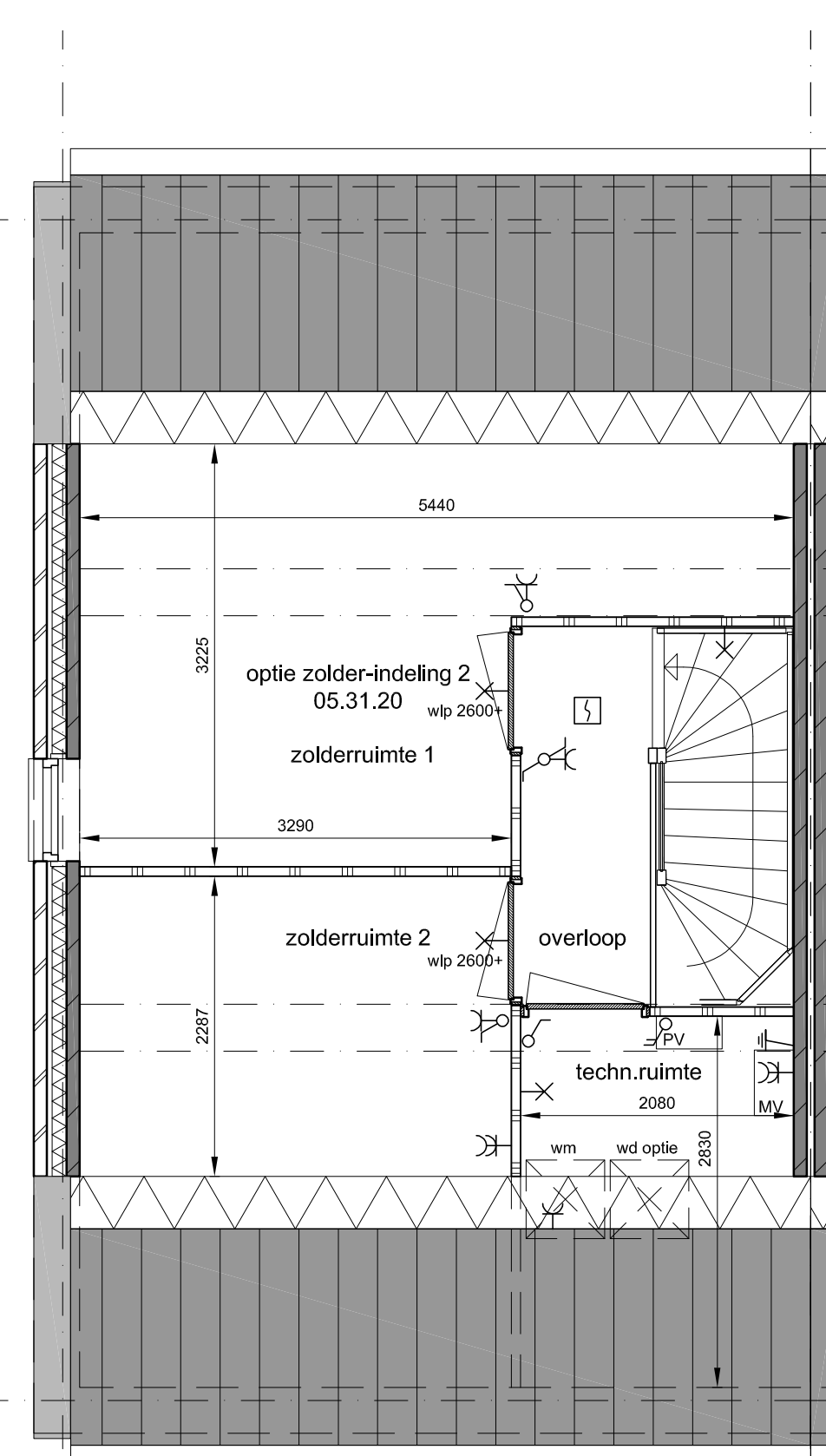
2e verdieping optie zolderindeling 2
