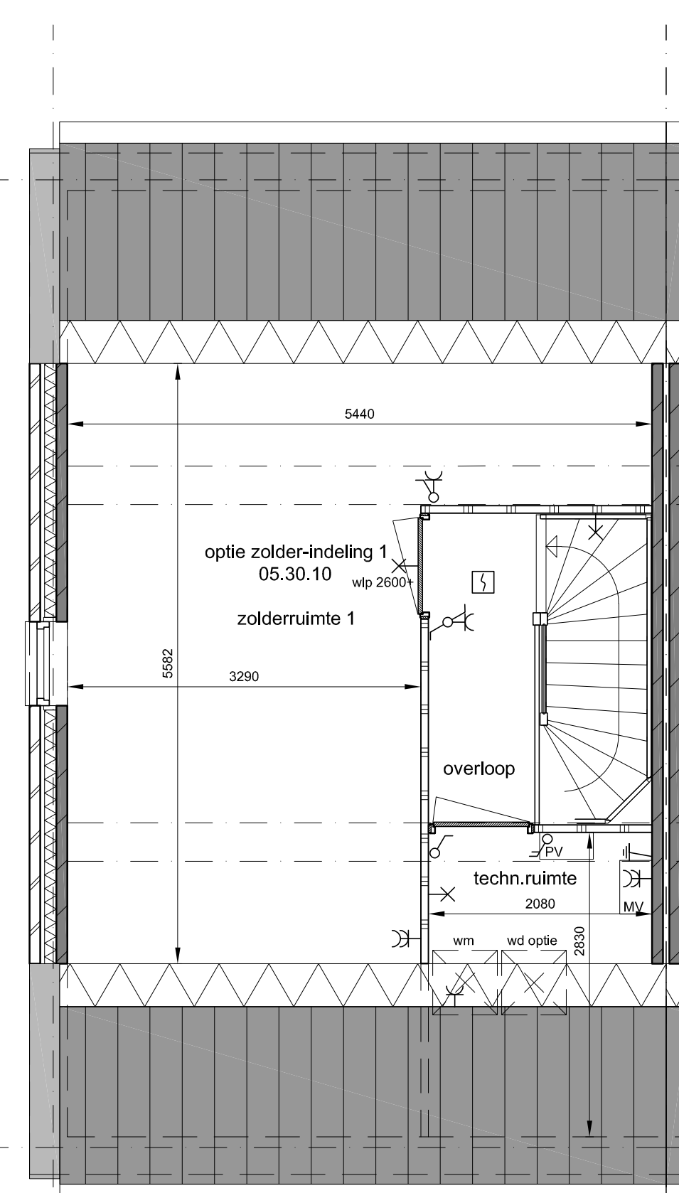
2e verdieping optie zolderindeling 1
