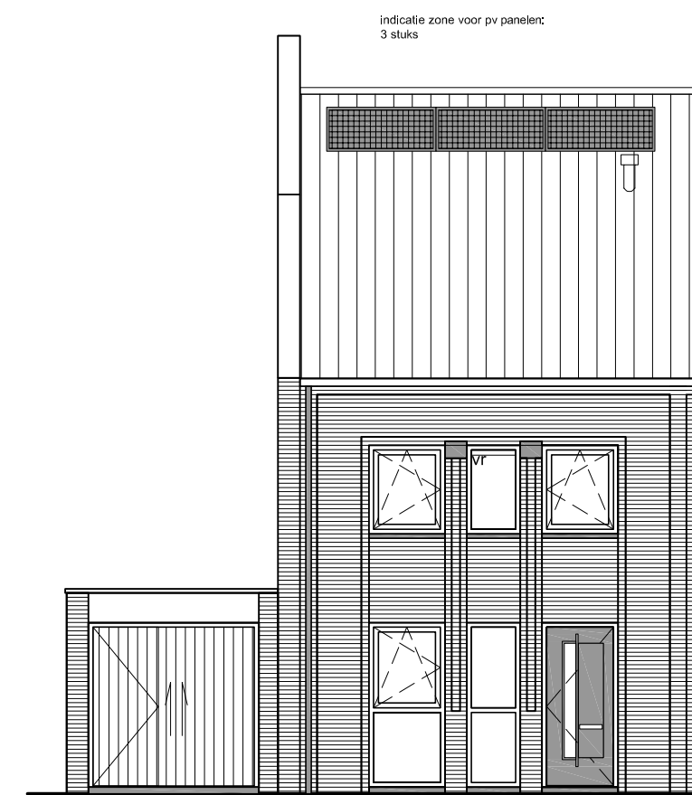
optie loopdeur in kanteledeur voorgevel
