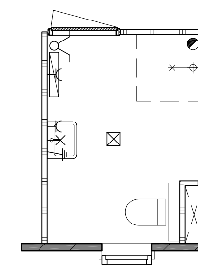
badkamerindeling 2
