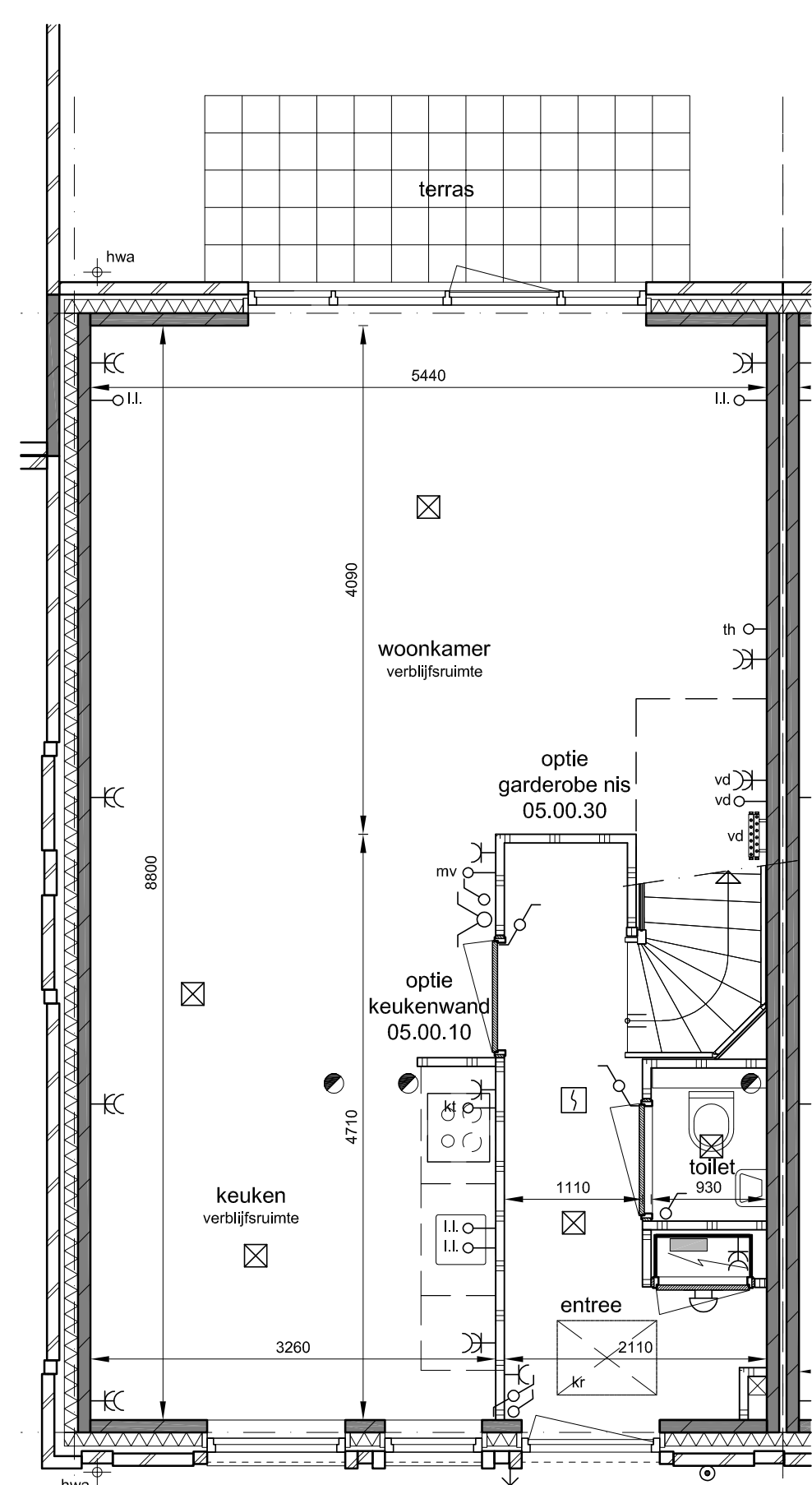
begane grond optie 75cm garderobe nis optie keukenwand
