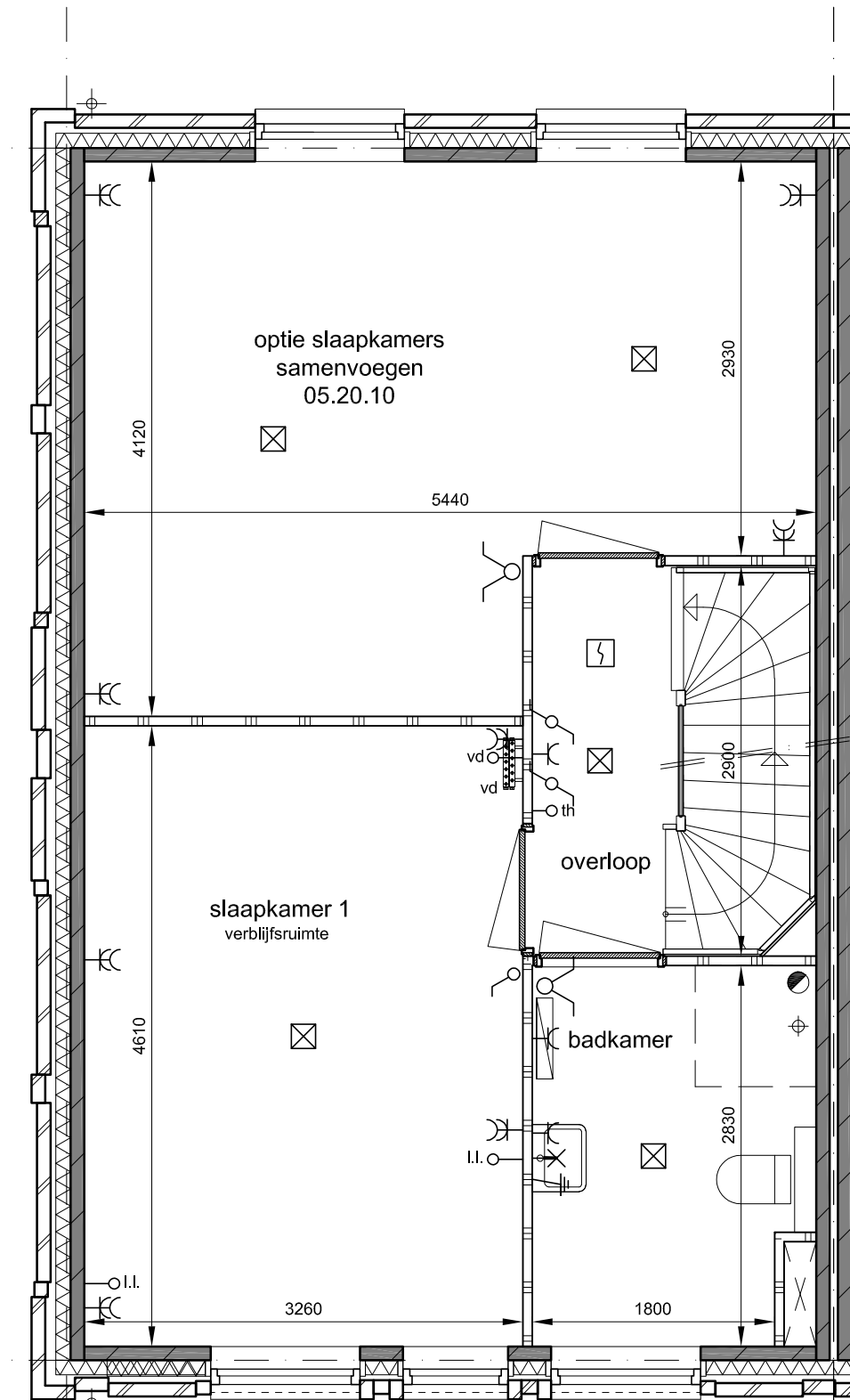
1e verdieping optie slaapkamer 2 en 3 samenvoegen deur achter
