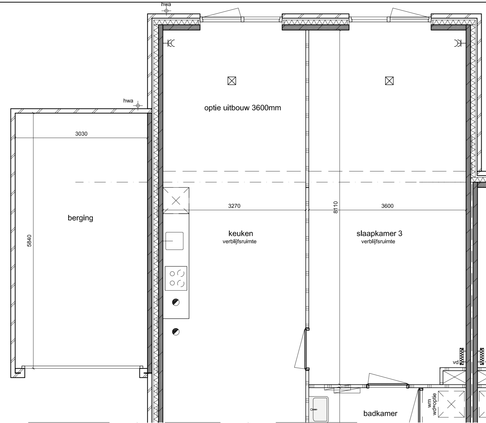
deelplattgrond uitbreiding 3600mm
