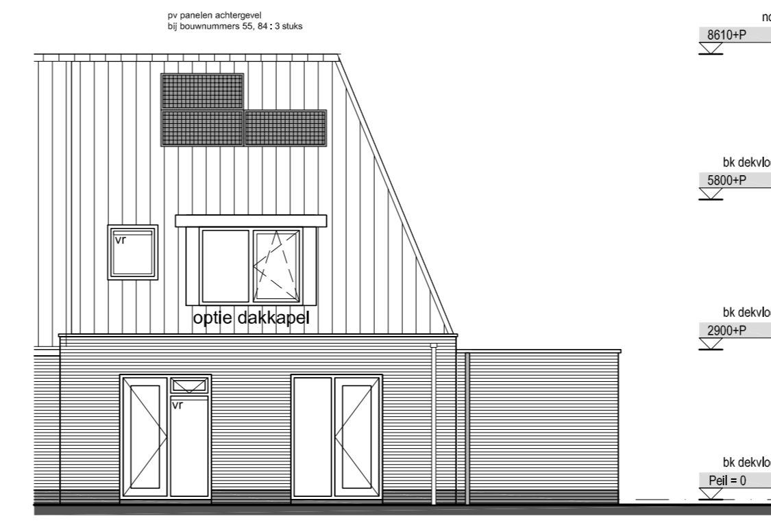
achtergevel optie uitbouw 2400mm
