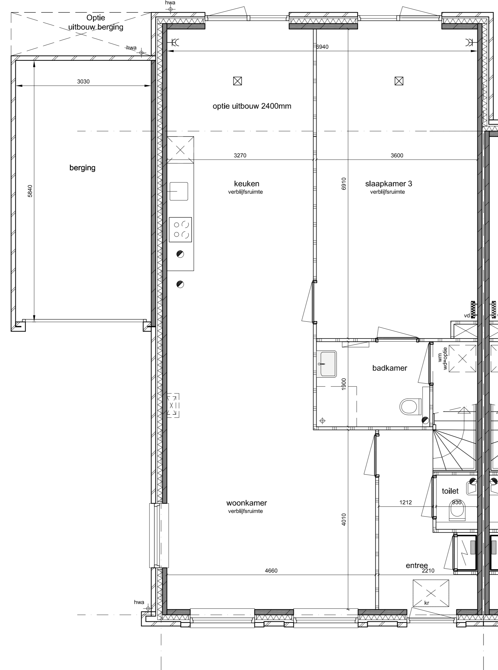
begane grond optie uitbouw 2400mm optie uitbreiding berging
