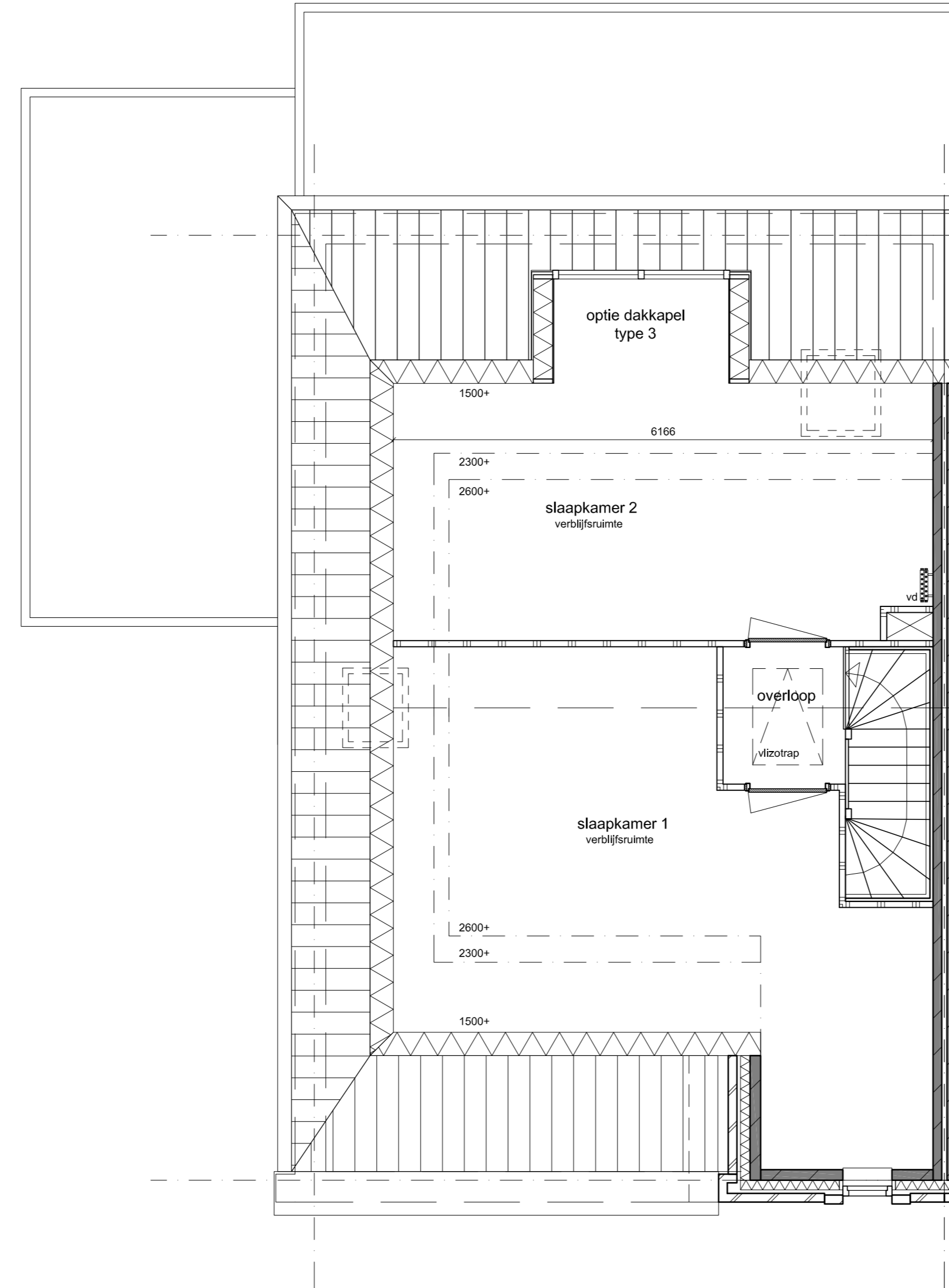
1e verdieping optie dakkapel aan achterzijde
