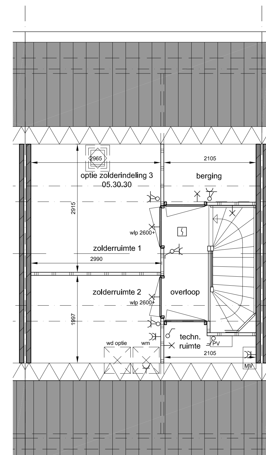
2e verdieping
