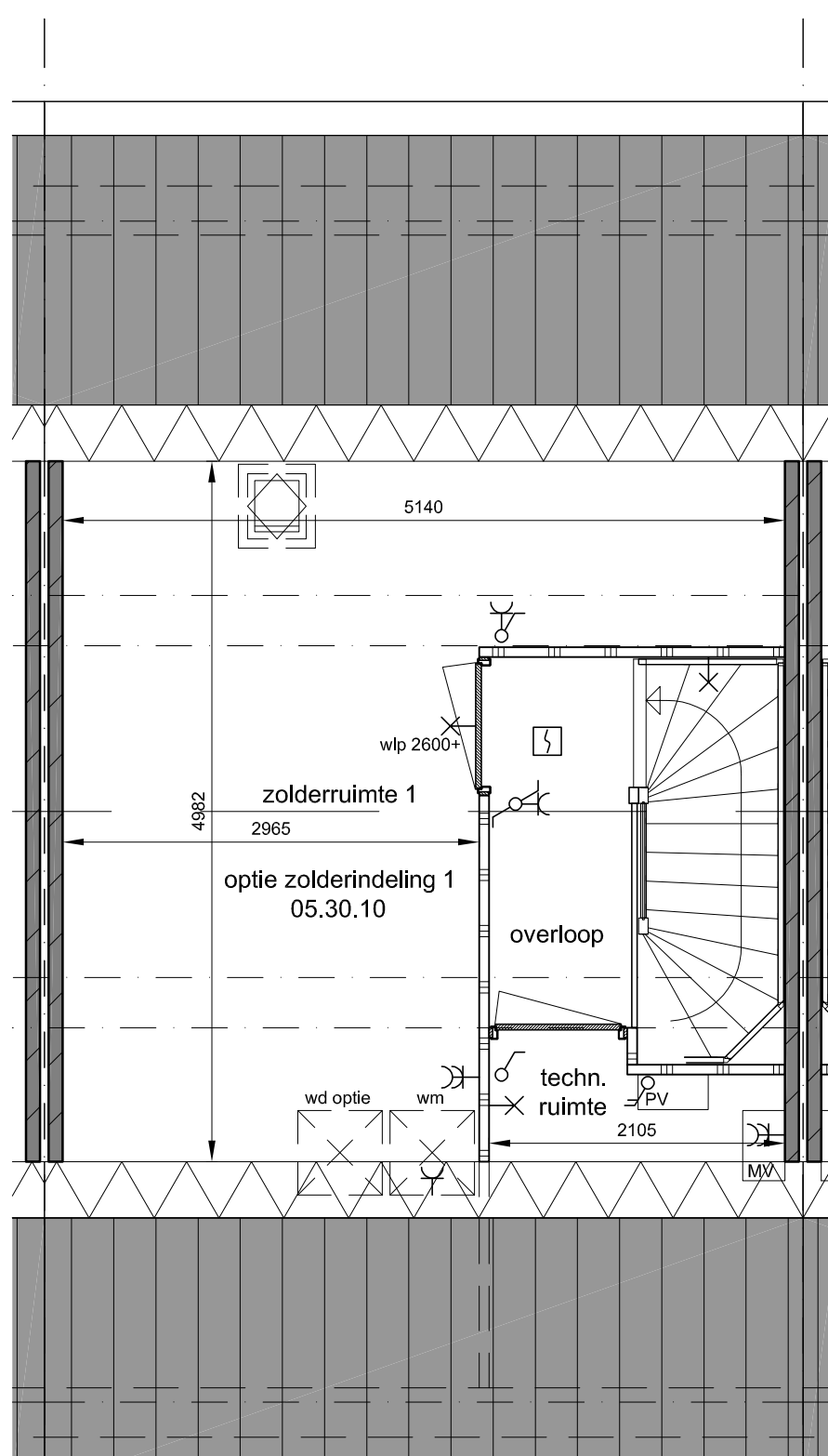
2e verdieping
