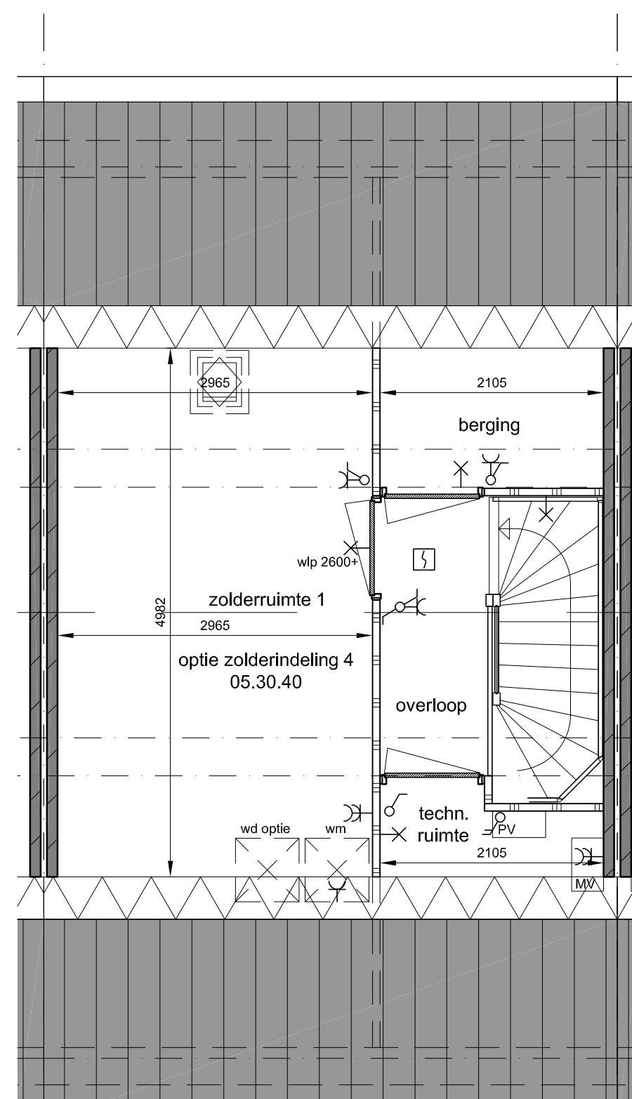
2e verdieping
