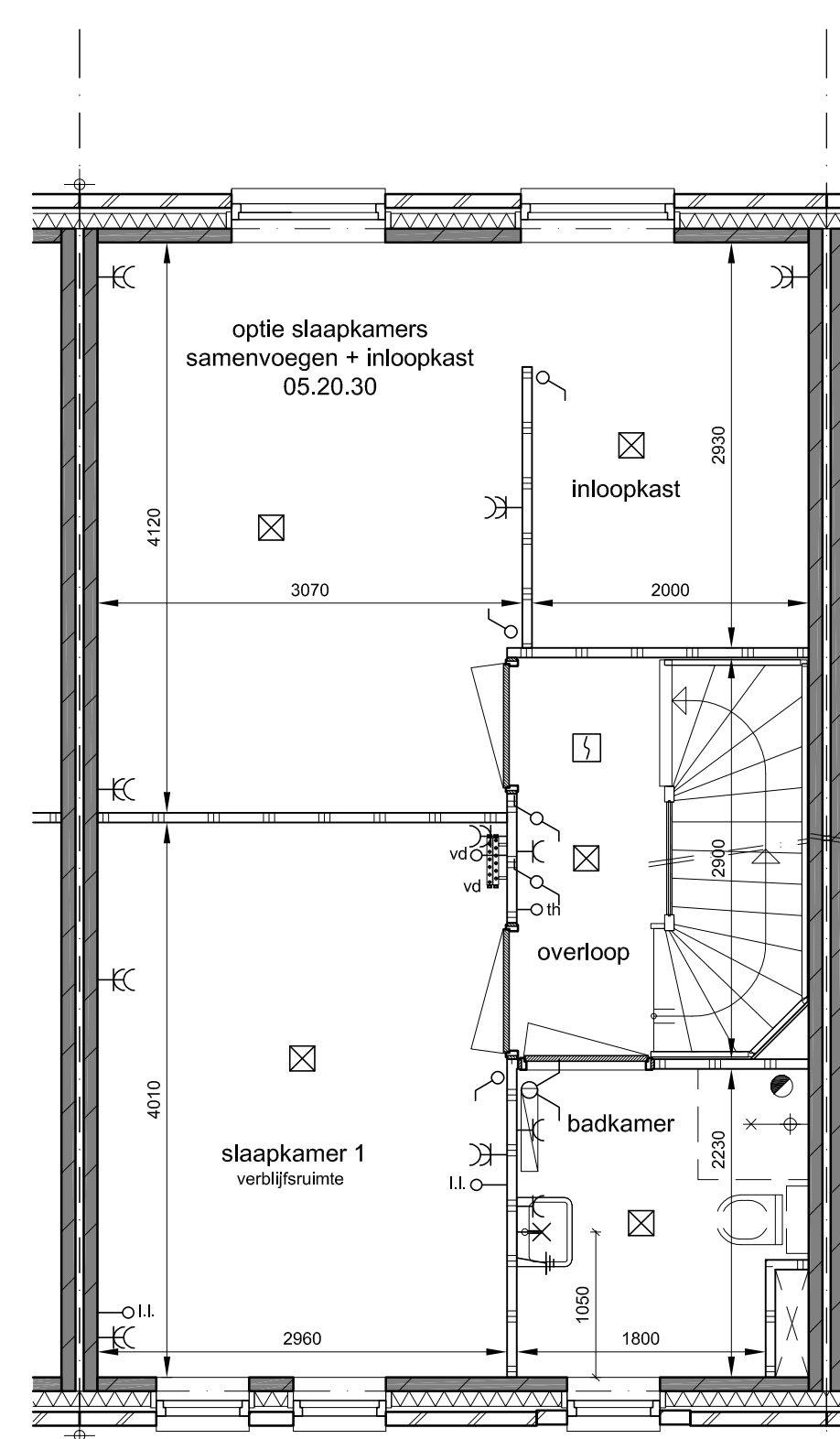
1e verdieping
