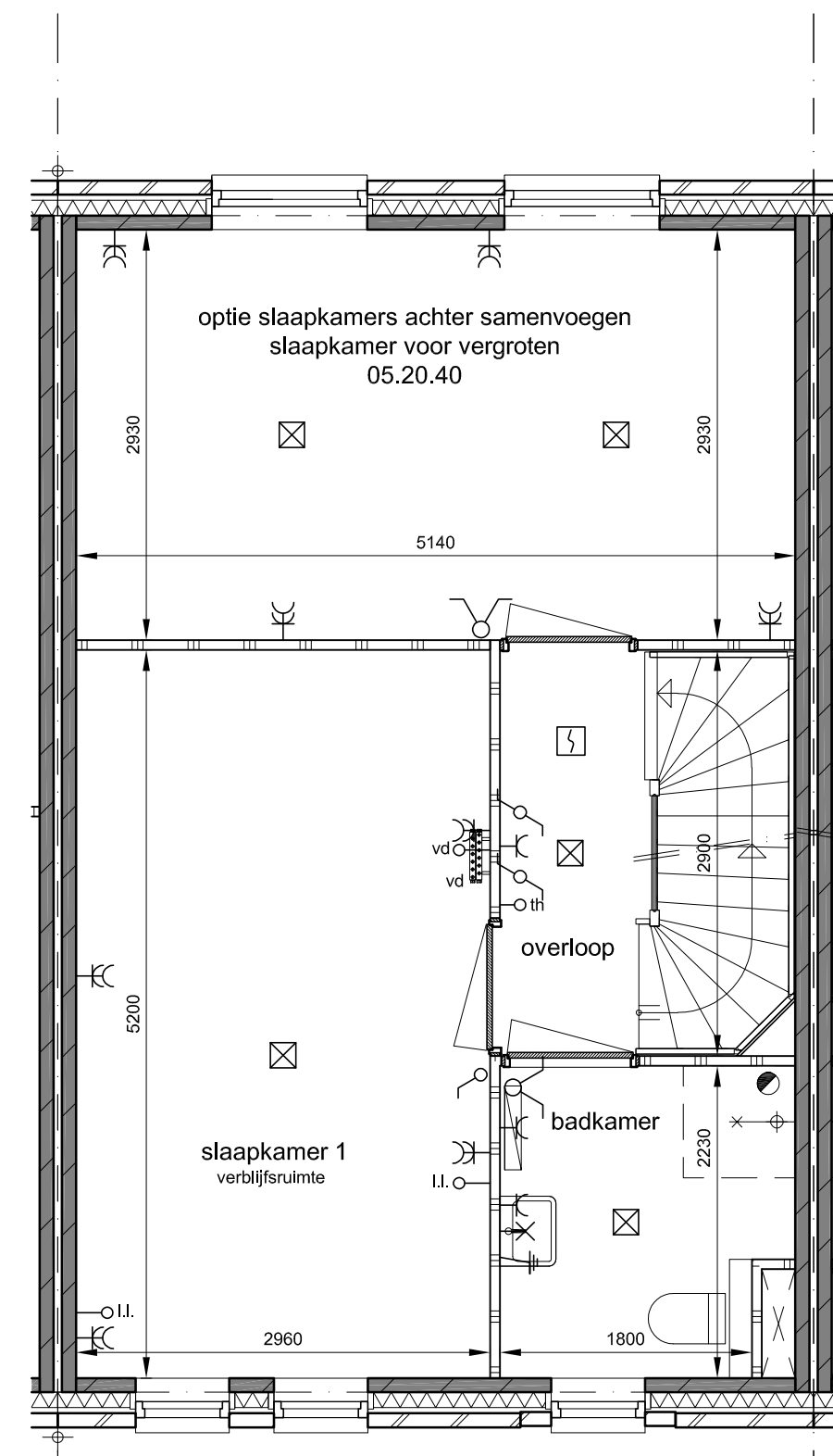
1e verdieping
