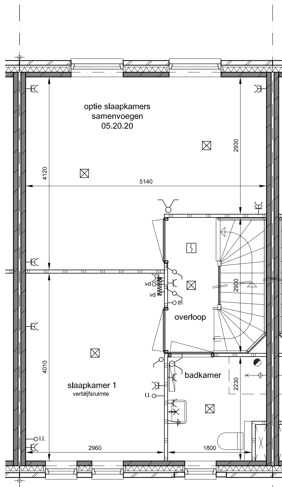
1e verdieping
