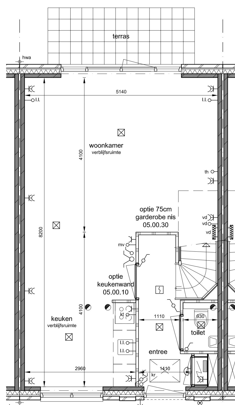
begane grond
