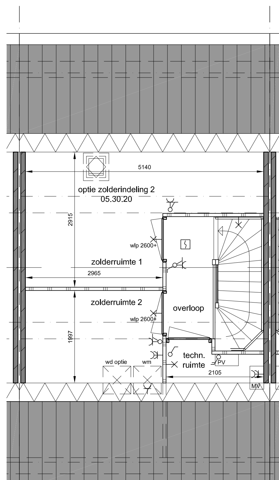
2e verdieping
