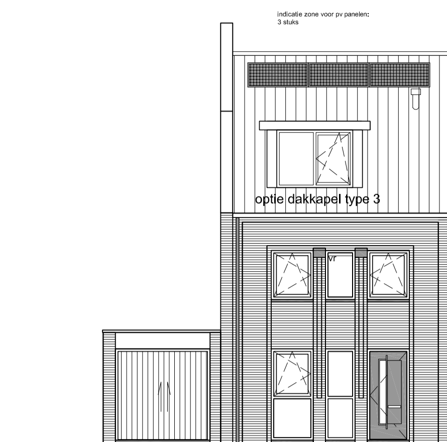
voorgevel
